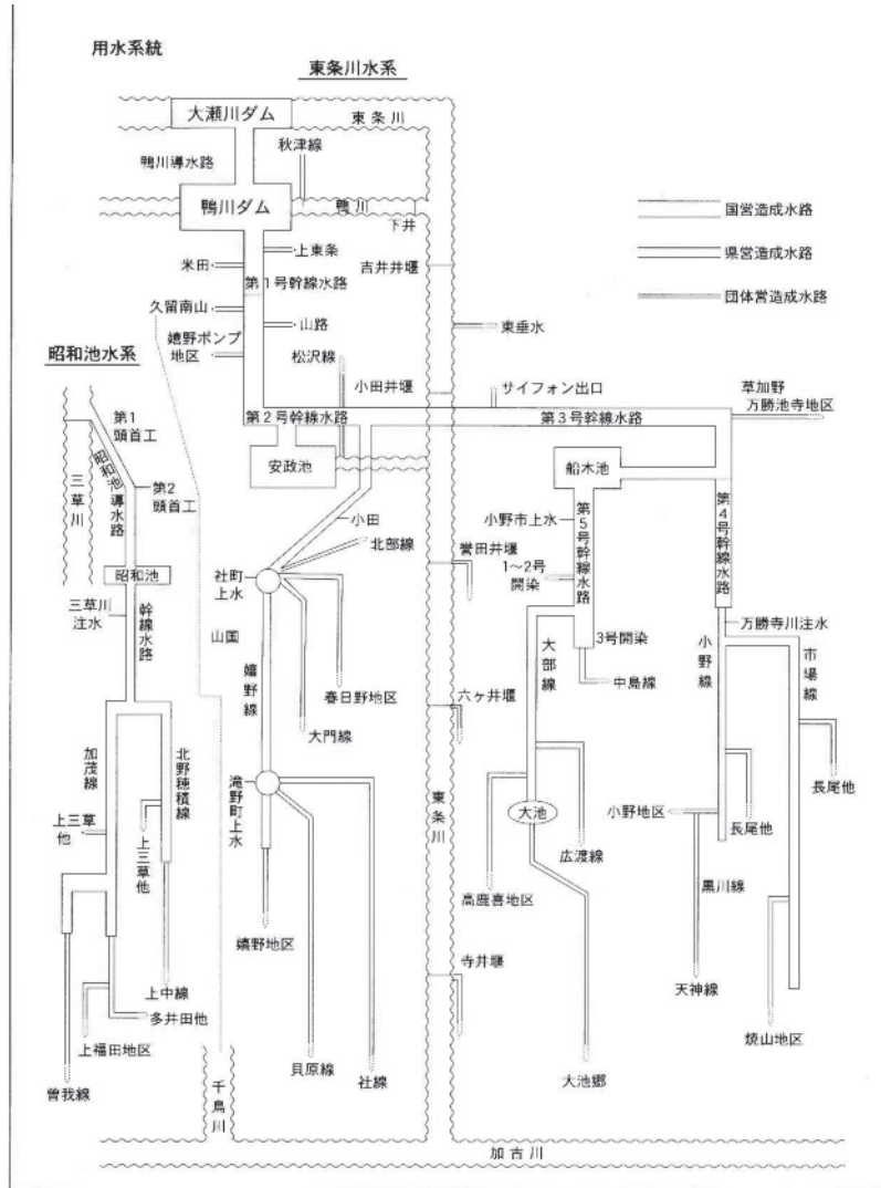
鴨川ダム用水系統図
